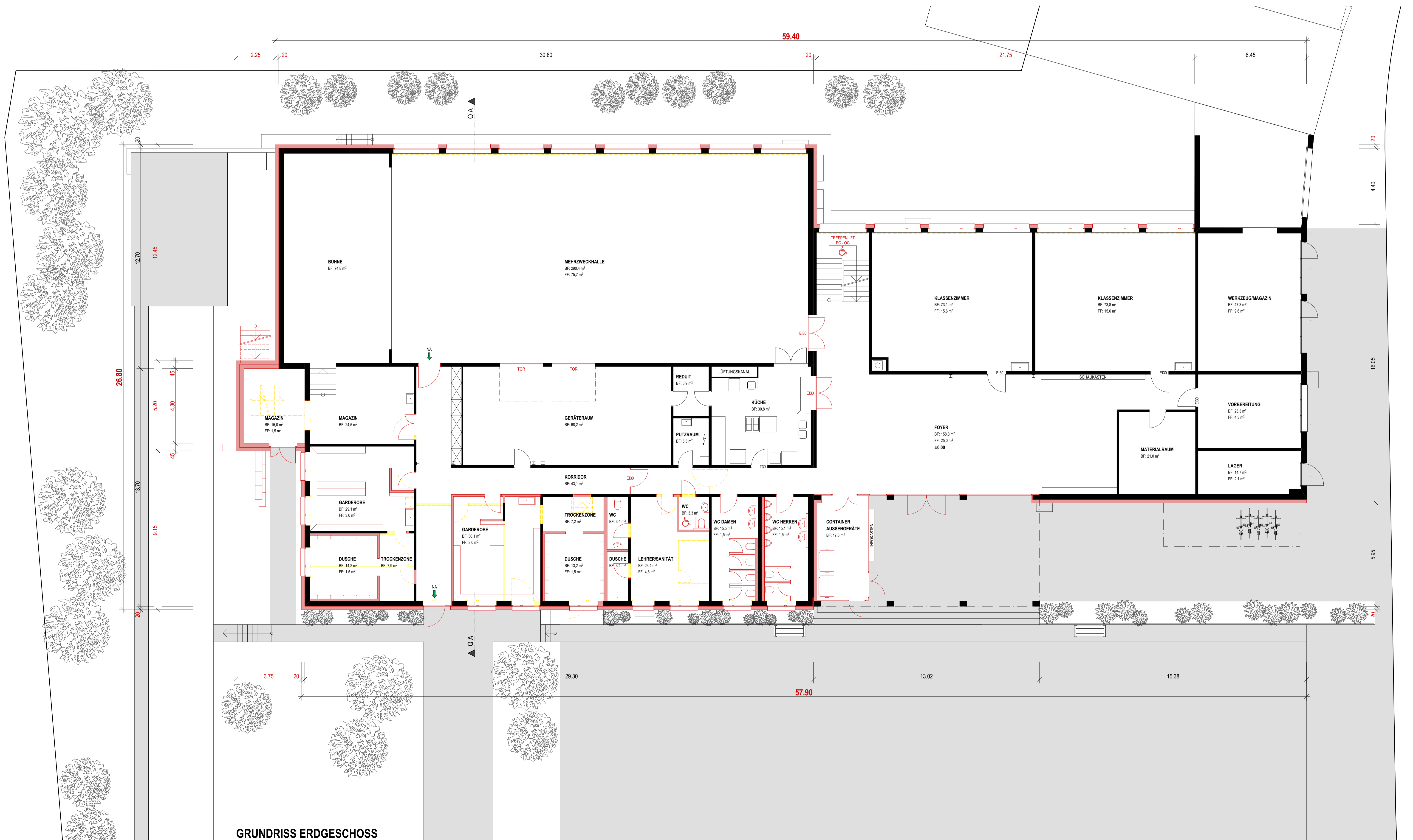
GRUNDRISS ERDGESCHOSS
