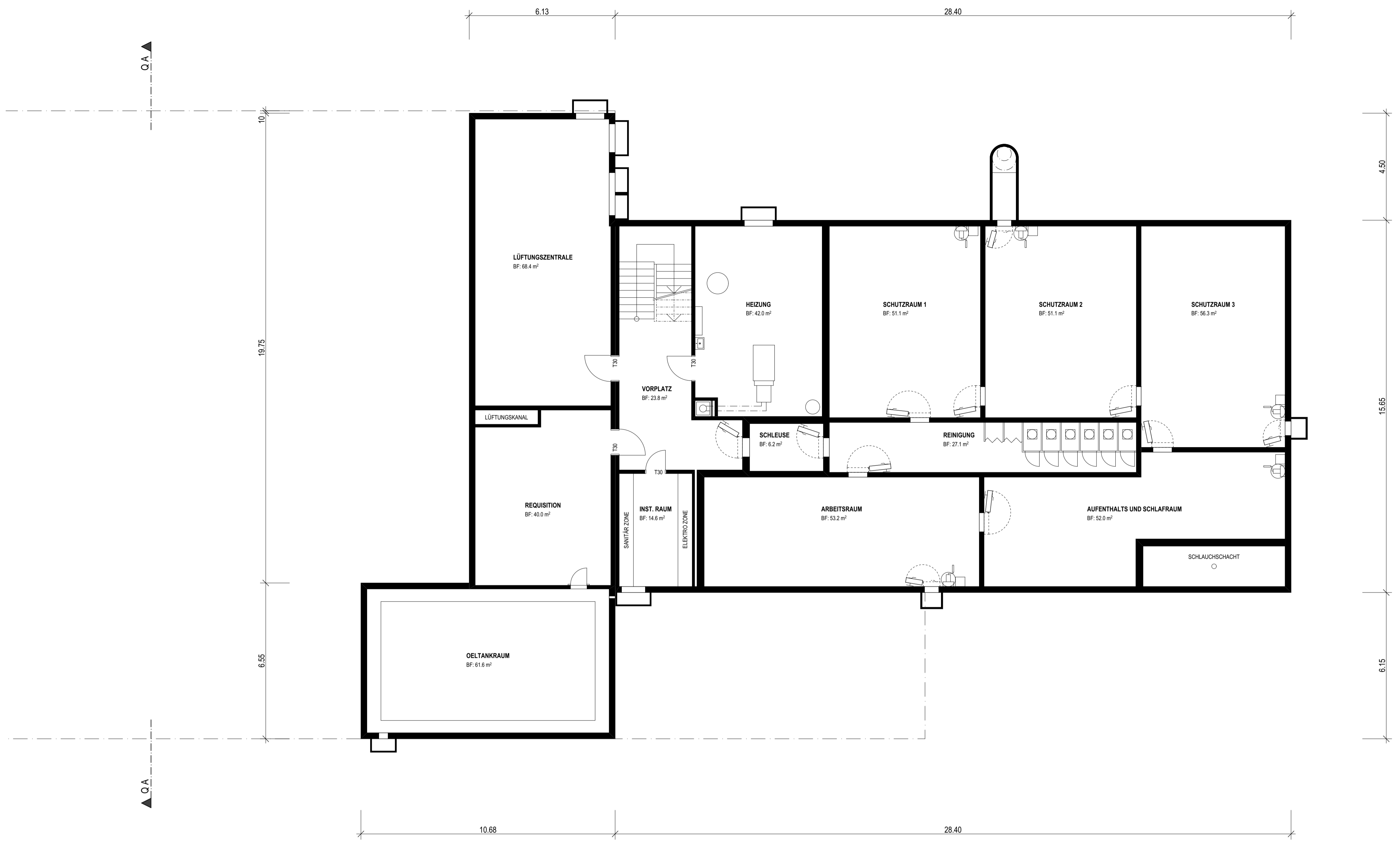
GRUNDRISS UNTERGESCHOSS
