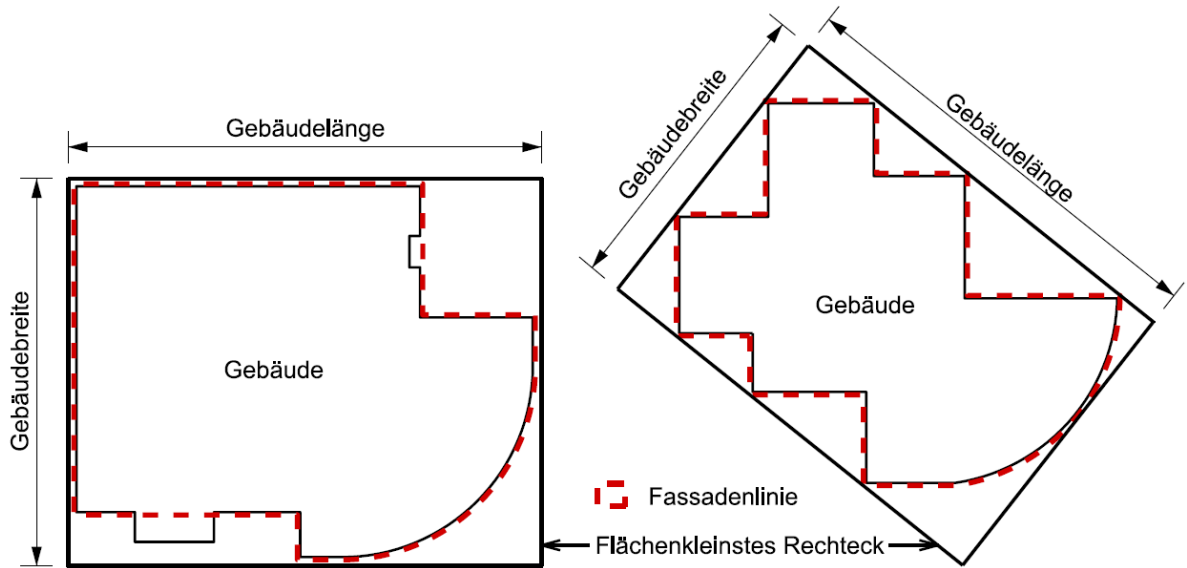
Figur zu Ziffer 4.1 Gebäuelänge, 4.2 Gebäudebreite
