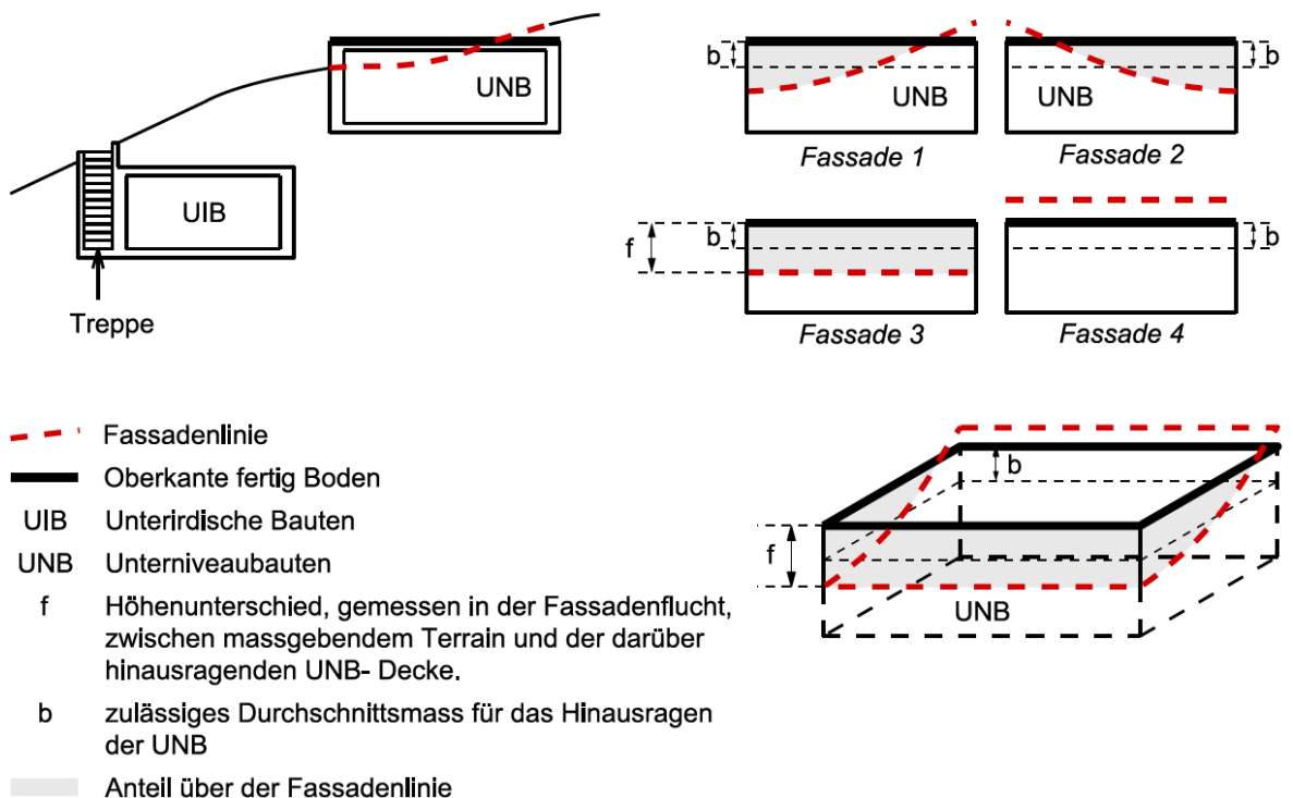
Figur zu Ziffer 2.4 Unterirdische Bauten, 2.5 Unterniveaubauten
